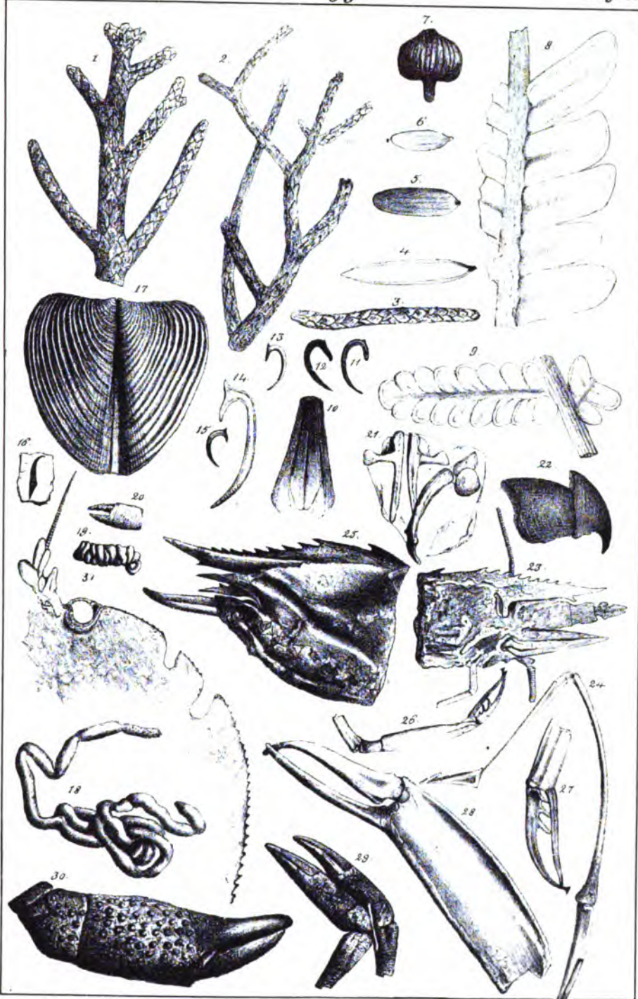
Quenstedt, Succa .
